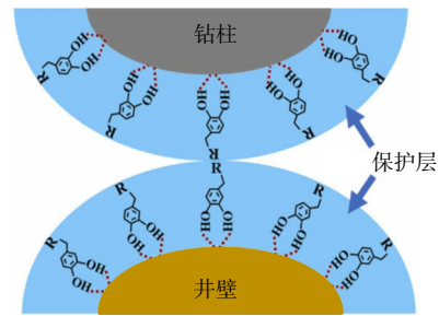
图 3 邻苯二酚在钻井液中的润滑机制
