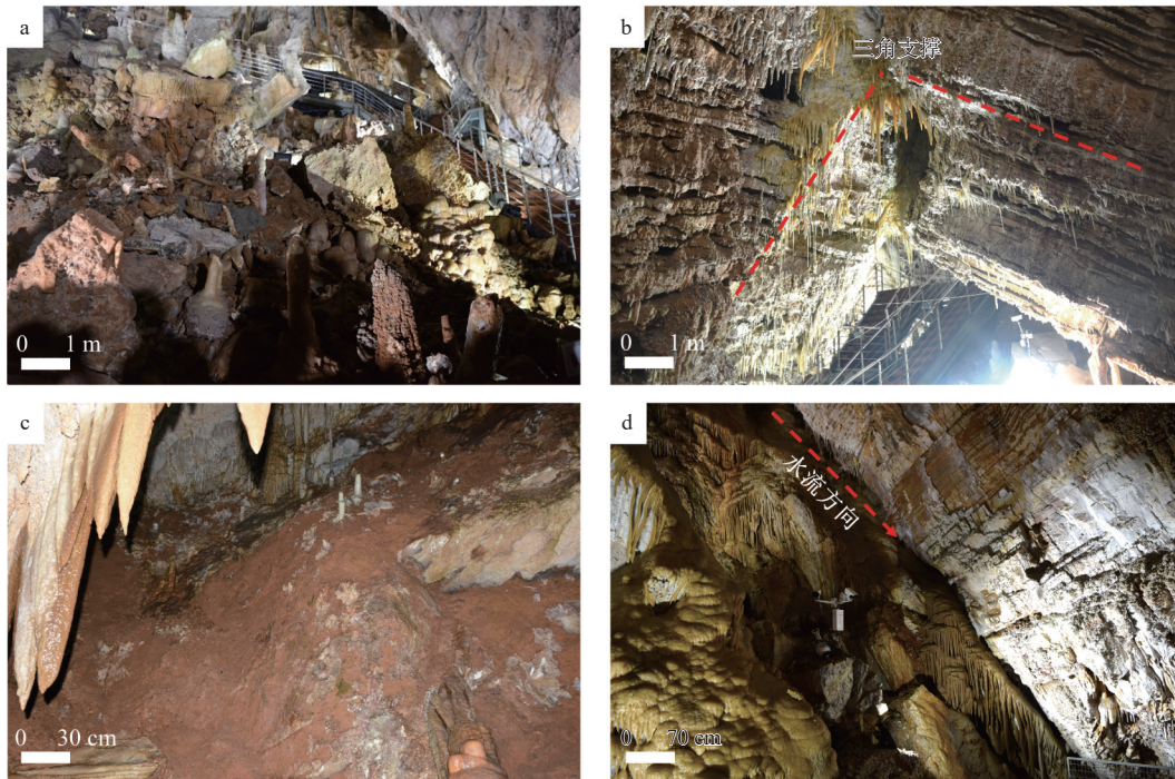
a—大厅中央崩塌的钟乳石；b—顶部的三角形支撑；c—灌入的红色古土壤；d—偏红色钟乳石
