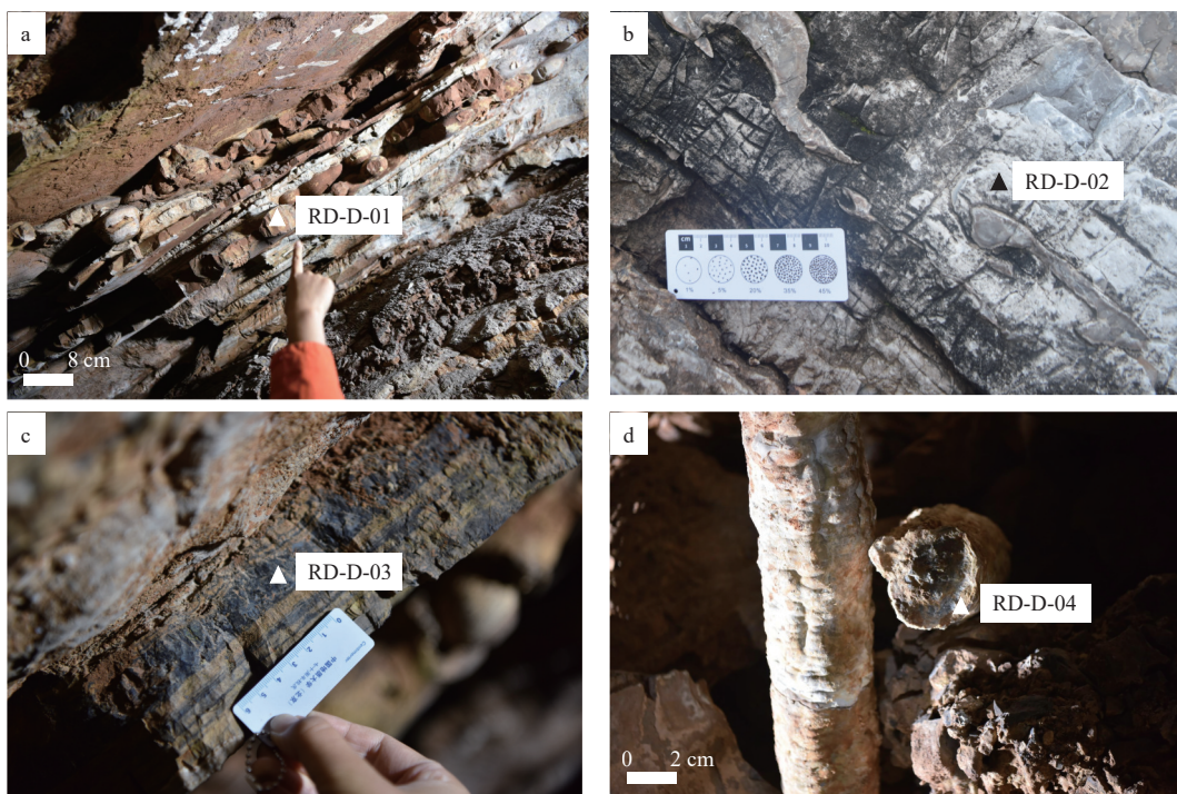
a—燧石团块; b—白云岩; c—灰岩; d—钟乳石
