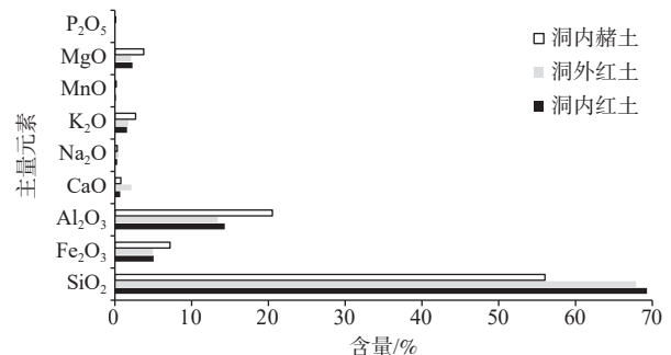
图 6 兴隆溶洞内外红土以及洞内赭土的主量元素地球化学特征
