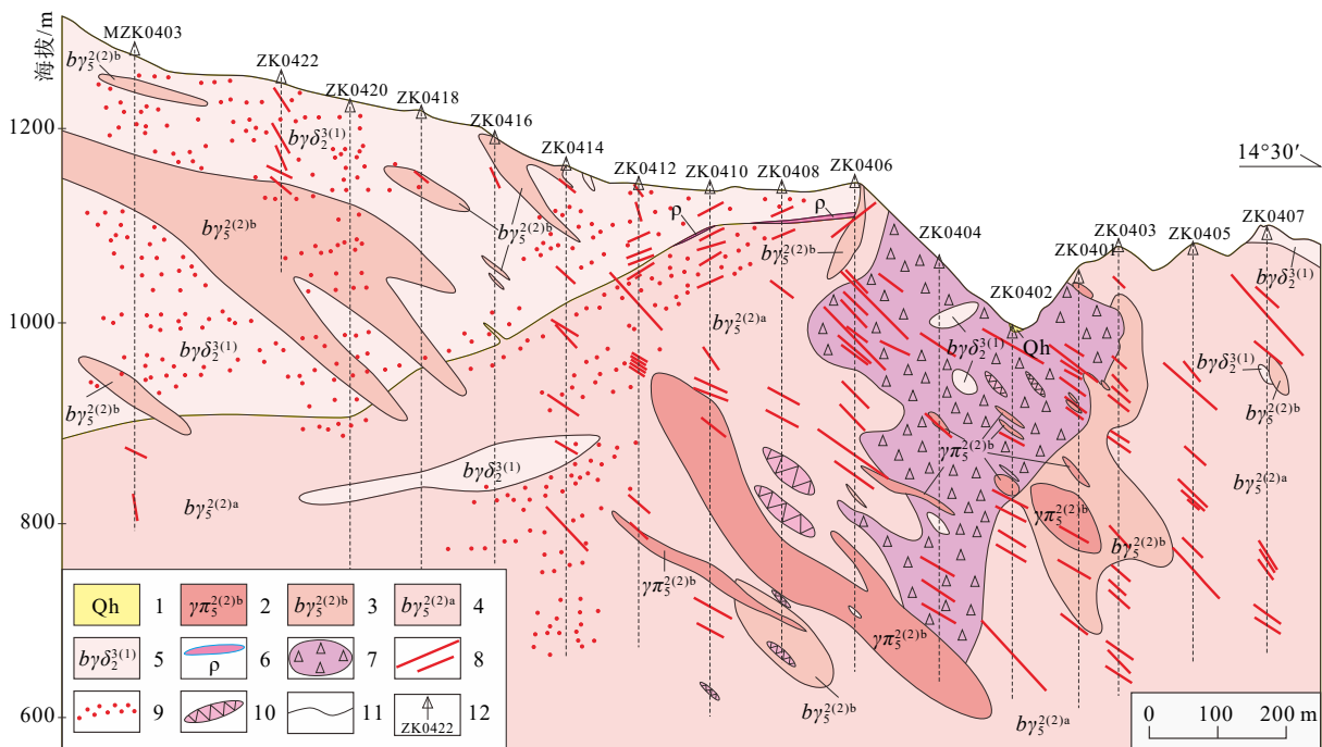
1—全新统; 2—燕山早期第二阶段花岗岩; 3—燕山早期第二阶段细粒黑云母花岗岩; 4—燕山早期第二阶段似斑状黑云母花岗岩; 5—晋宁期中粗粒黑云母花岗岩闪长岩; 6—似伟晶岩; 7—热液隐爆角砾岩型矿体; 8—石英大脉型钨矿体; 9—细脉浸染型钨矿体; 10—无矿石英团块、石英脉带; 11—地质界线; 12—钻孔及编号
