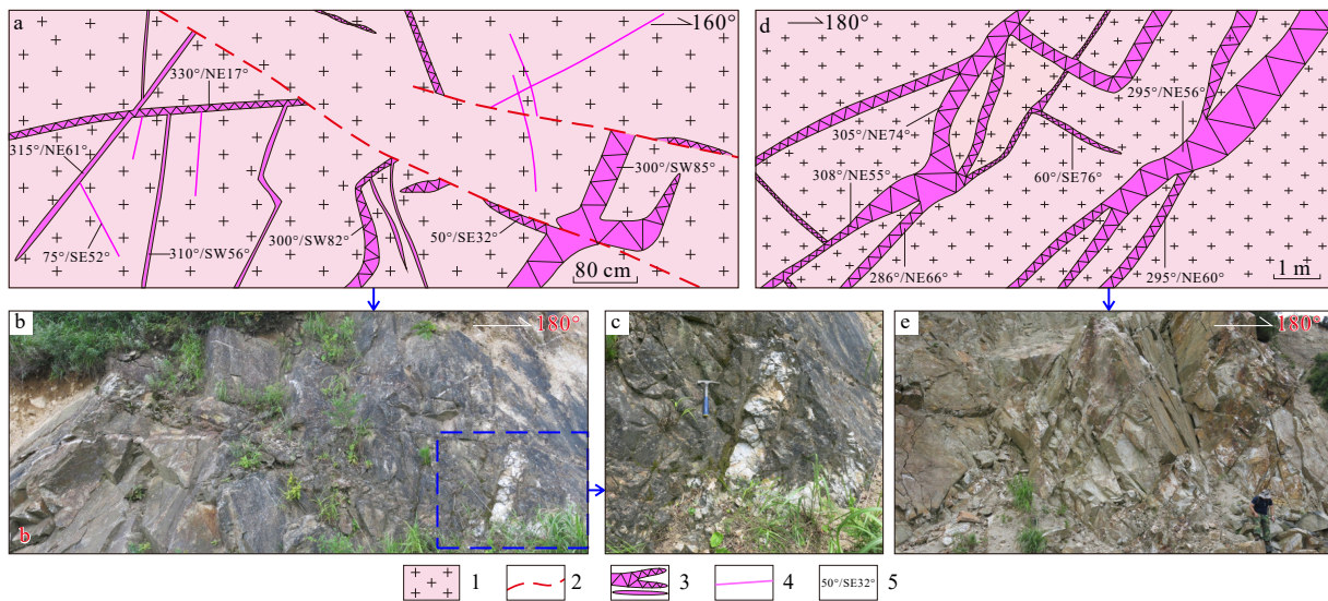
1—晋宁期花岗岩; 2—晚期裂隙/断裂; 3—含钨石英脉(4~40 cm); 4—含钨石英细脉(1~3 cm); 5—产状 a—中等倾角南倾中细含钨石英脉, 矿区东南部, D12-2点; b—剖面 a 对应的照片; c—照片 b 的局部放大; d—中等倾角北倾粗大含钨石英脉, 矿区中北部, D5-3点; e—剖面 d 对应的照片, 含钨石英脉最宽达 80 cm
