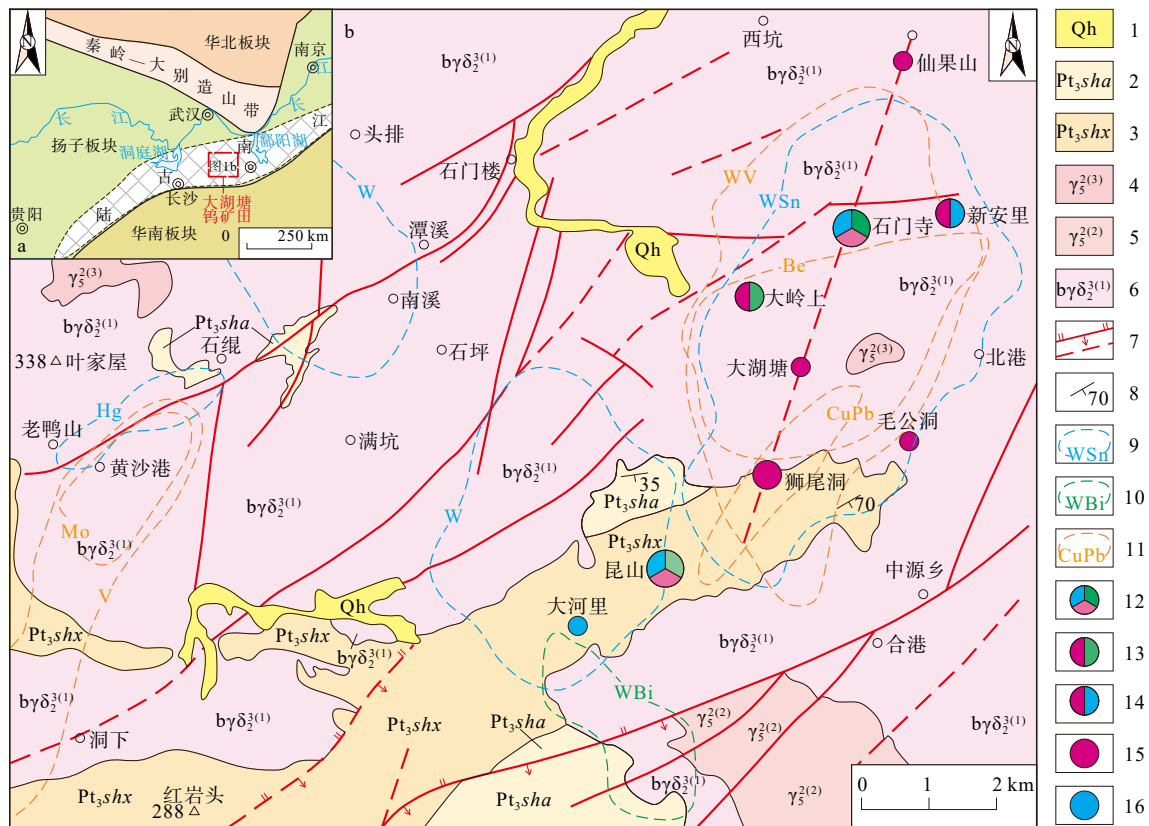
1—全新统；2—新元古界双桥山群安乐山组千枚状变凝灰质砂岩和绢云母千枚岩；3—新元古界双桥山群修水组变凝灰质砂岩和粉砂质板岩；4—燕山晚期花岗岩；5—燕山早期花岗岩；6—晋宁晚期黑云母花岗闪长岩；7—断层；8—产状；9—重砂扩散晕；10—土壤测量分散晕；11—岩石测量原生晕；12—钨铜钼矿床；13—钨铜矿床；14—钨钼矿床；15—钨矿床；16—钼矿床
