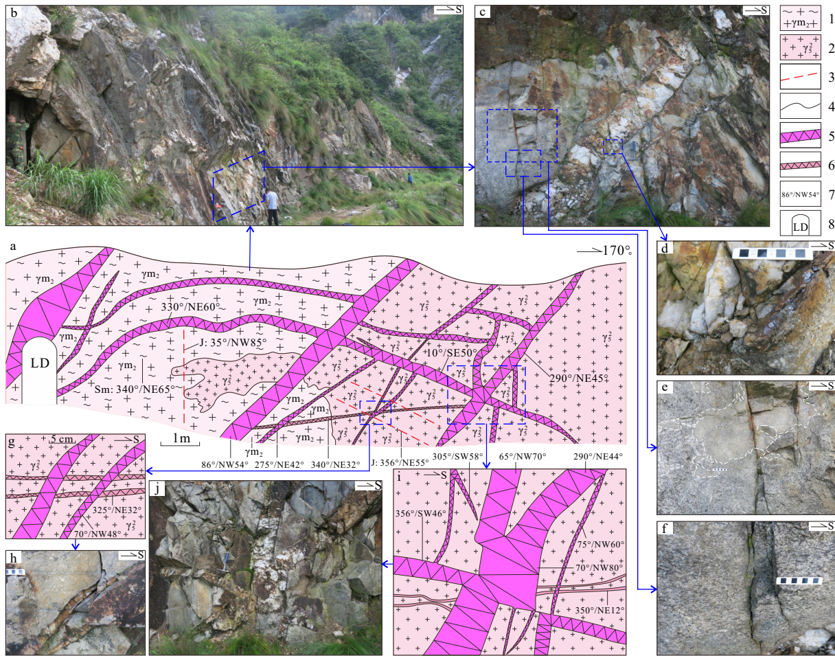
1—片麻状花岗岩；2—中细粒花岗岩；3—无矿节理裂隙；4—地质界线；5—含钨石英脉；6—早期无矿石英细脉；7—产状；8—老硐 a—含钨石英脉素描，矿区中北部，D02点；b—剖面a对应的照片；c—图片b中部偏北侧局部放大，示走向近东西向中等倾角北倾的含钨石英大脉；d—图片c的局部放大，示含钨石英脉边部发育辉钼矿；e—图片c的局部放大，示含钨石英脉的围岩燕山期细粒花岗岩侵入在晋宁期片麻状粗粒花岗岩闪长岩中；f—图片c的局部放大，示含钨石英脉围岩晋宁期片麻状粗粒花岗岩闪长岩；g—剖面a中部局部放大素描，示北东东向中等倾角北倾含钨石英脉，穿切早期无矿石英细脉；h—剖面g对应的照片；i—剖面a的南部局部放大素描，示多个产状含钨石英脉同时贯入结晶，穿切早期无矿石英细脉；j—剖面i对应的照片
