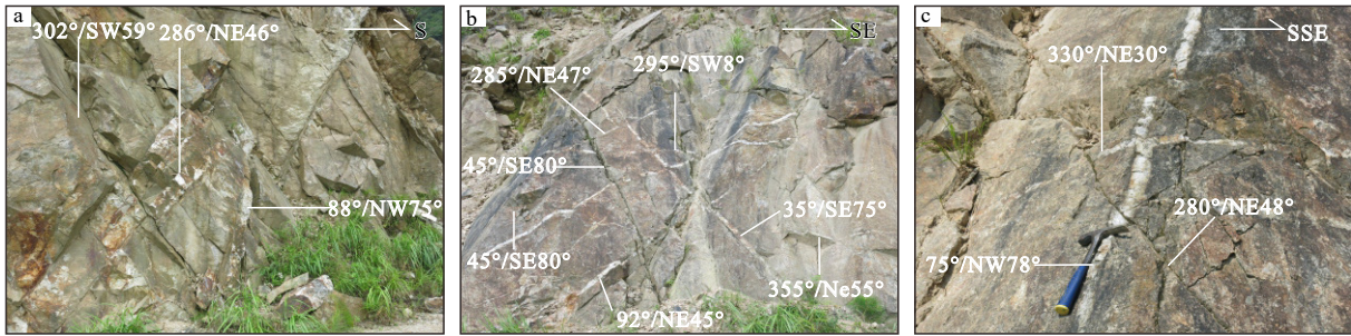
a—含矿裂隙与不含矿裂隙, D06-2点; b—含矿裂隙与不含矿裂隙, D14-1点; c—含矿裂隙与不含矿裂隙, D14-2点
