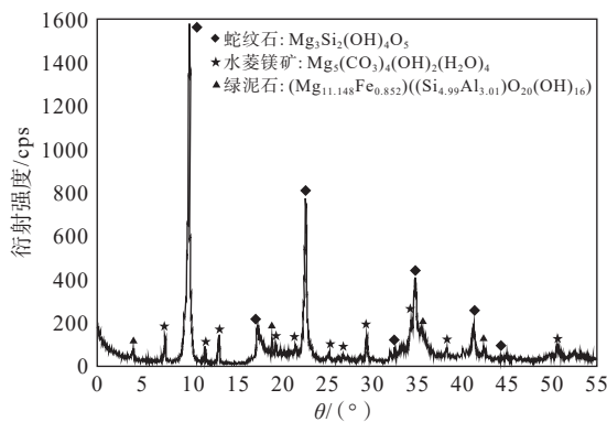
(a) 蚀变岩滑带土黏土XRD定量测试结果
