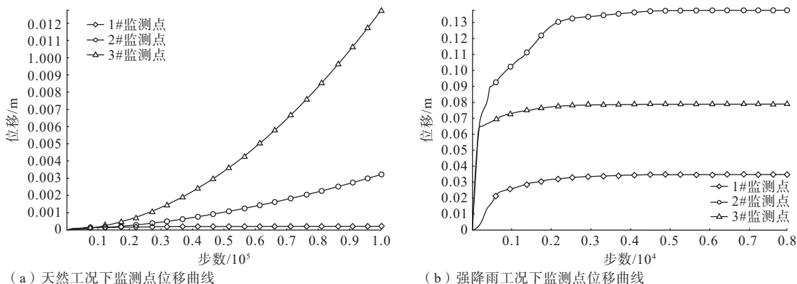
图 9 不同工况下监测点位移曲线
