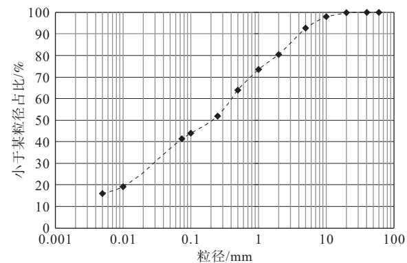
(b) 蚀变岩滑带土粒径分布曲线
