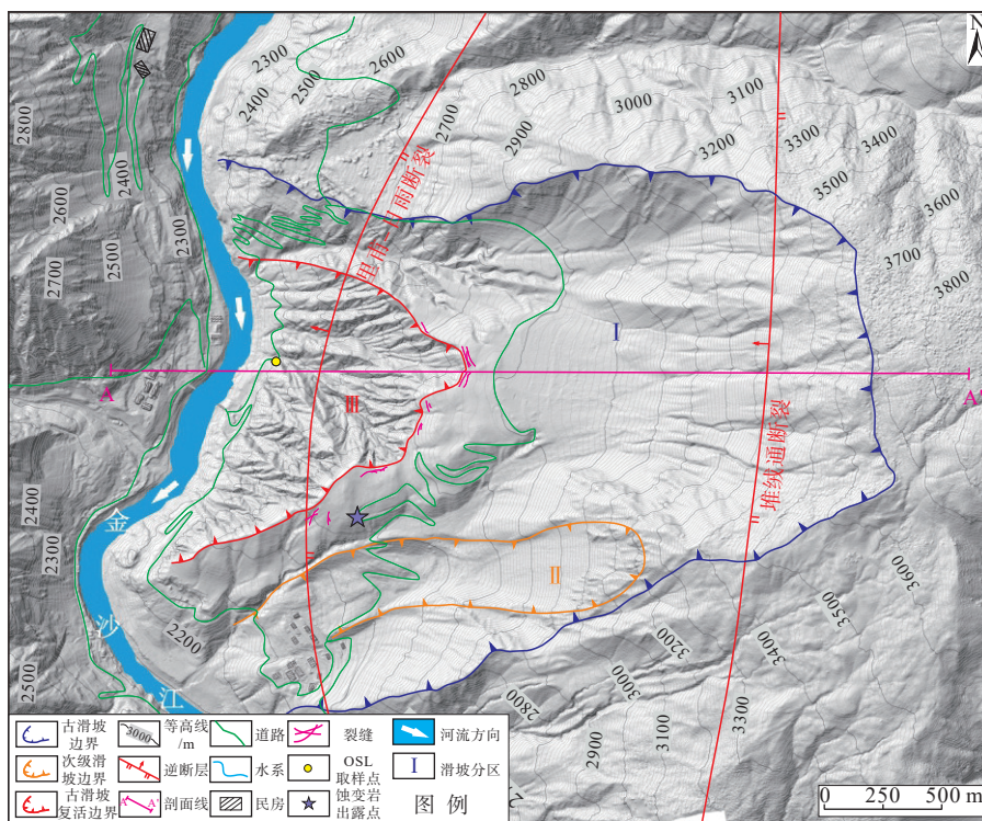
图 3 堆绒通滑坡平面分区图
