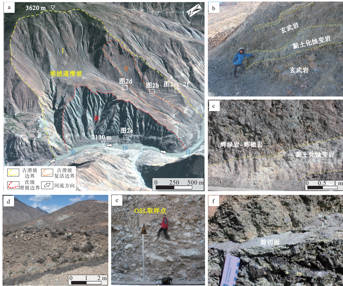
a—滑坡全景(底图来自 google earth); b—滑坡中部黏土化蚀变岩条带; c—滑坡左侧公路旁出露的黏土化蚀变岩条带; d—滑坡中部堆积块石特征(镜向北西); e—滑坡前缘发育的冲洪积阶地及光释光(OSL)测年取样位置; f—滑坡左侧蛇绿岩中发育的黏土化蚀变岩滑带
