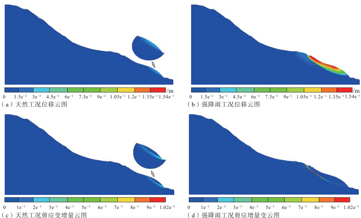
图 8 不同工况下位移云图与应变增量云图
