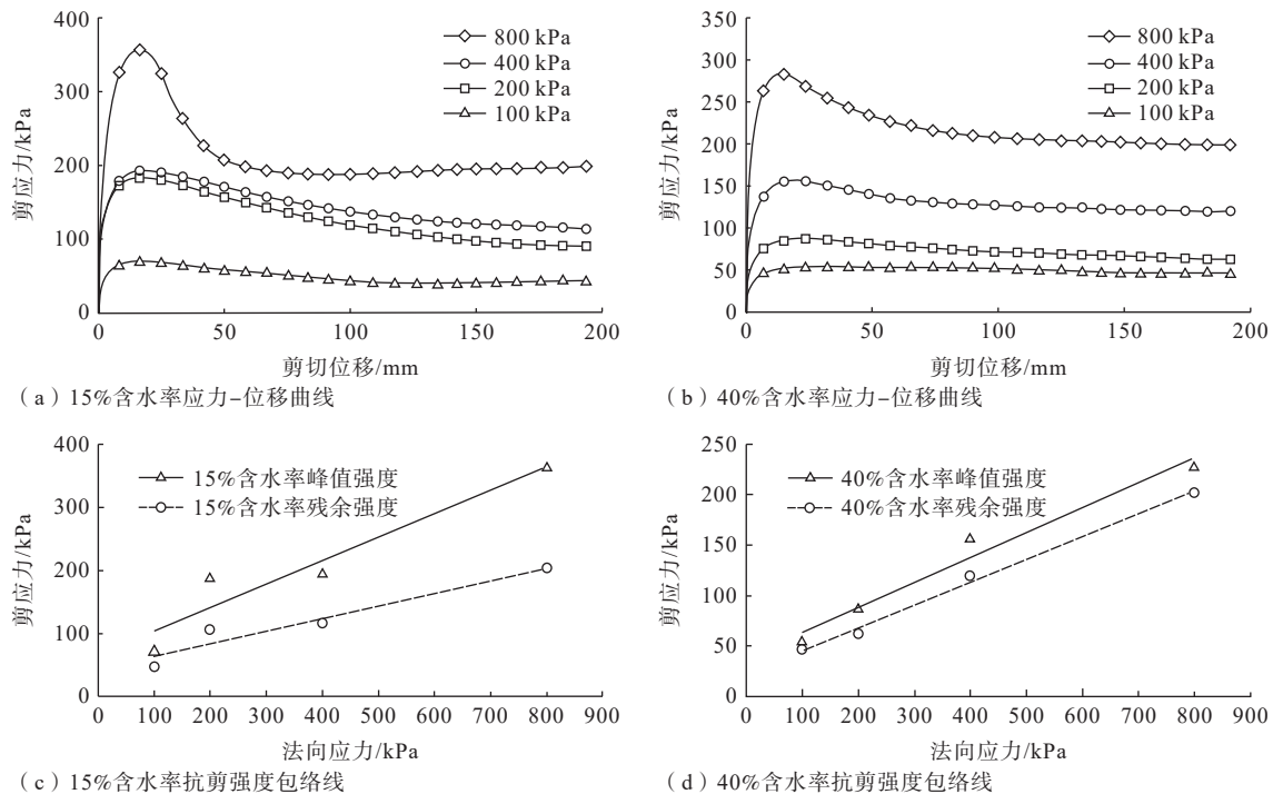
图6 黏土化蚀变岩应力-位移关系曲线及强度包络线
