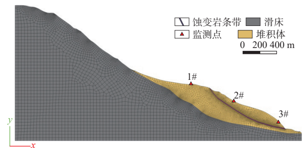
图 7 堆绒通滑坡地质概化模型
