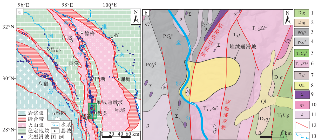
a—三江构造缝合带大型滑坡分布图; b—堆绒通滑坡及周边地质略图
