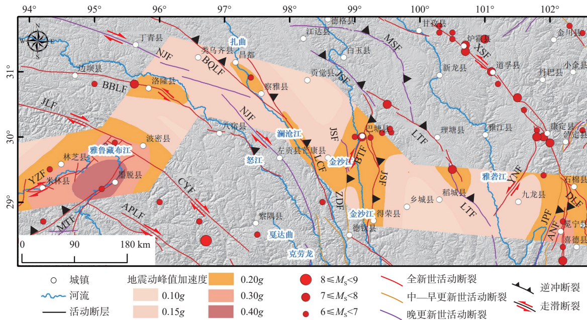
MTF—墨脱断裂; APLF—阿帕龙断裂; YZF—雅鲁藏布江断裂; CYF—察隅断裂; JLF—嘉黎断裂; BBLF—边坝—洛隆断裂; NJF—怒江断裂; LCF—澜沧江断裂; JSF—金沙江断裂; MSF—麦宿断裂; BQLF—巴青—类乌齐断裂; XSF—鲜水河断裂; LTF—理塘断裂; YNF—玉农希断裂; ANF—安宁河断裂; DLF—大凉山断裂; JPF—锦屏山断裂; ZDF—字嘎寺—德钦断裂
