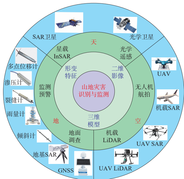
图 17 天-空-地一体化灾害识别、监测与预警技术体系 (据许强等, 2019 修改)
